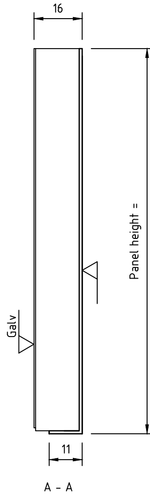
A - A
